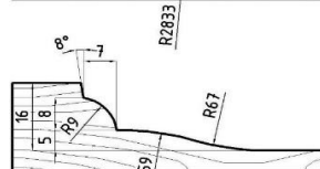
Филенка с ножами из стали 9ХС
